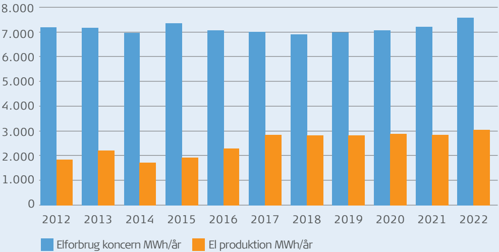
ELFORBRUG OG PRODUKTION – KONCERN MWH/ÅR
